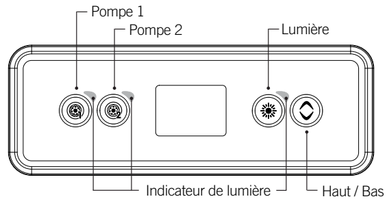
Modèle 2 pompes
